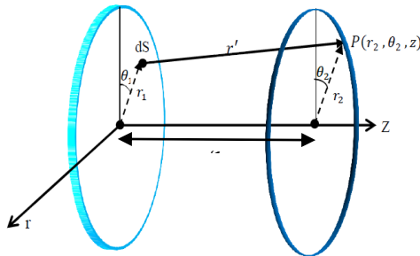
شکل ۱ نمایی از هندسه مورد استفاده الگوسازی در مختصات استوانه‌ای. دیسک سمت چپ تراگذار فراصدا، P(r_1, \theta_1, z) نقطه هدف برای تعیین فشار صوتی و dS عنصری از سطح بلور است.
