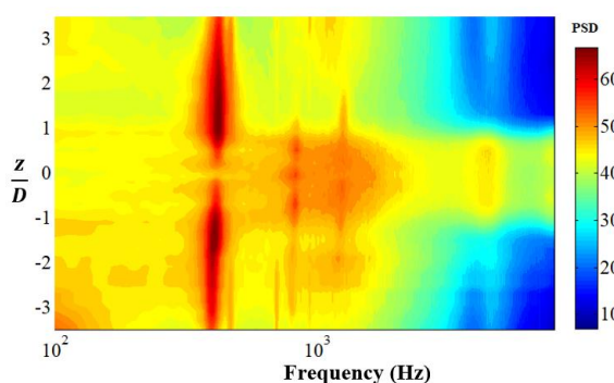
شکل ۲۲ کانتور چگالی طیف فشار کل در پایین دست استوانه در موقعیت L=2D (سرعت ۳۰ متر بر ثانیه).
