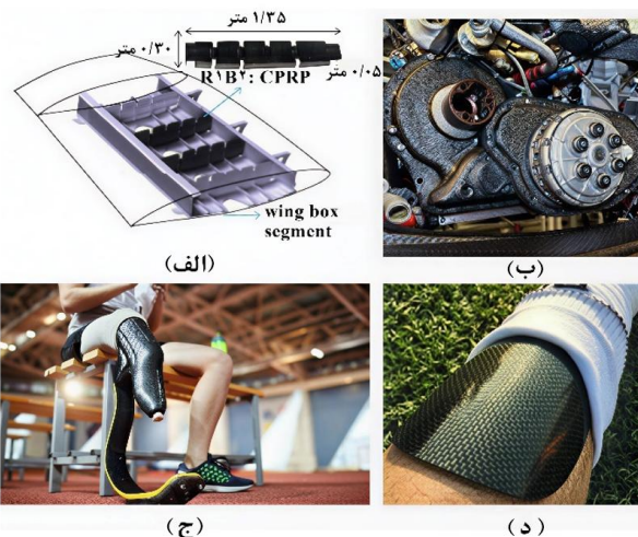
شکل ۲ کاربرد الیاف کربن در صنایع مختلف و کاربردهای خاص [۲۴-۲۸].
