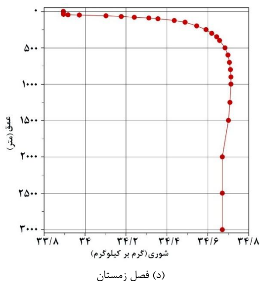
شکل ۴ تغییرات فصلی الگوی شوری نسبت به عمق در شرق قطب جنوب.
