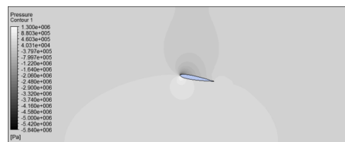
شکل ۸ توزیع فشار حول آونازکورت (هیدروفویل) در زاویه حمله ۱۰ درجه.
