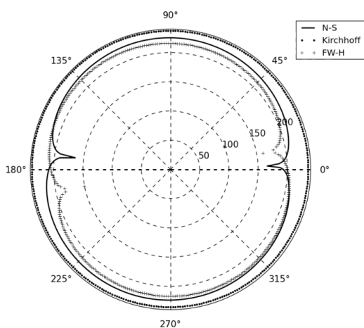
شکل ۷ نمودار تراز فشار صوتی روش‌های کرشهف، فوکز-ویلیامز و هاکینگز و ناویه-استوکس برای \frac{Z}{c} = 0.01 .
