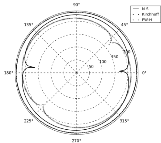
شکل ۸ نمودار تراز فشار صوتی روش‌های کرشلف، فوکز-ویلیامز و هاکینگز و ناویه-استوکس برای \frac{Z}{c} = 0.076 .
