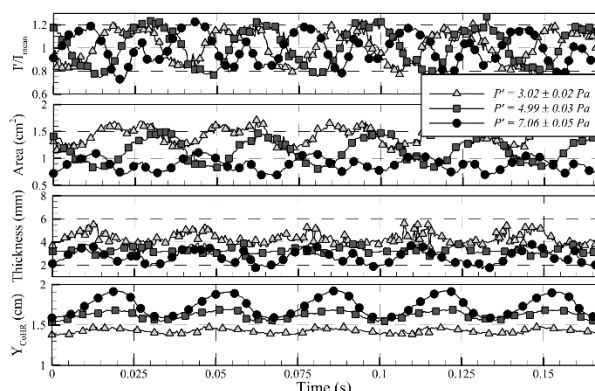
شکل ۹ جابه‌جایی مرکز سطح تابش، سطح، ضخامت و نرخ رهائش حرارت لحظه‌ای شعله در بسامد ۳۰ هرتز و دامنه‌های فشار مختلف.
