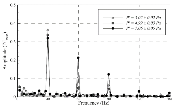
شکل ۱۰ تبدیل فوریه سریع نرخ رهائش حرارت لحظه‌ای شعله در بسامد ۳۰ هرتز و دامنه‌های فشار مختلف.
