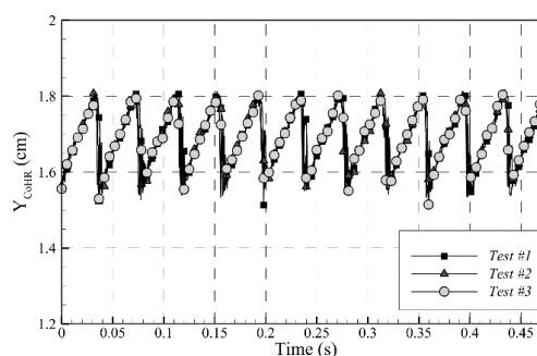
شکل ۸ جابه‌جایی مرکز سطح تابش شعله در سه آزمون تکرار در بسامد ۲۵ هرتز و دامنه فشار ۵ پاسکال.
