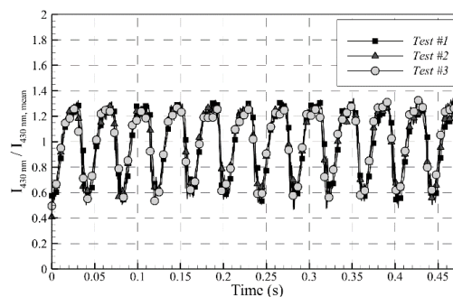
شکل ۹ شدت تابش بی‌بعد شده رادیکال سی‌اچ‌اِستار در سه آزمون تکرار در بسامد ۲۵ هرتز و دامنه فشار ۵ پاسکال.
