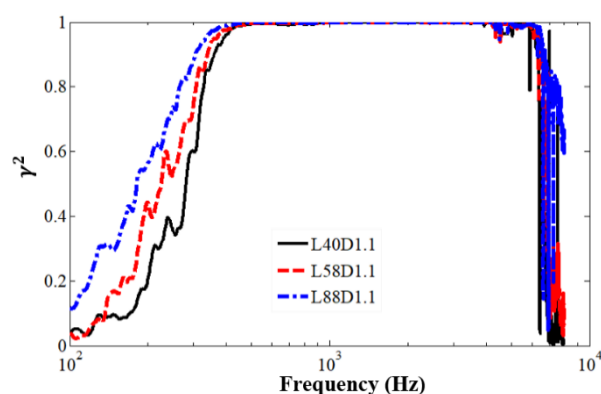
شکل ۵ مقایسه نمودار همدوسی به ازای تغییر طول لوله کاوشگر.
