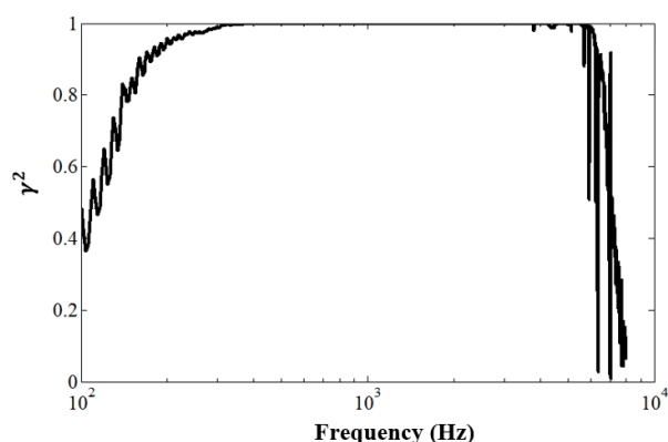
شکل ۱۲ نمودار تابع همدوسی بین سیگنال دریافتی کاوشگر و مرجع.
