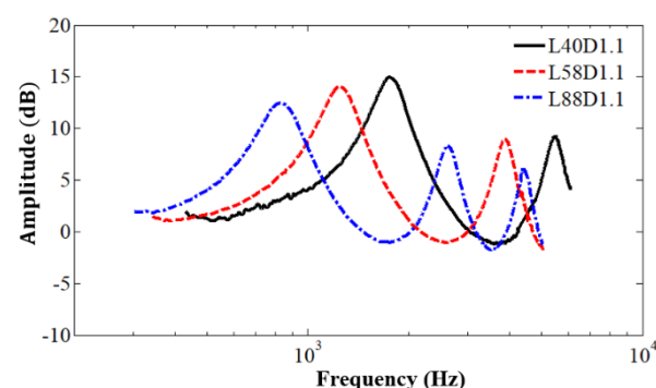
شکل ۶ مقایسه نمودار تغییرات دامنه تابع انتقال سامانه به ازای تغییر طول لوله ی کاوشگر.
