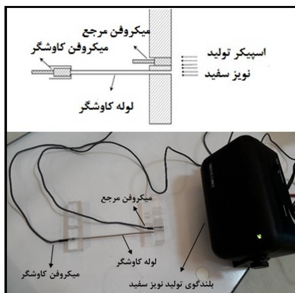
شکل ۳. شماتیک و تصویری از چینش تعیین تابع انتقال سامانه.
