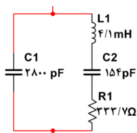
شکل ۵ مدار معادل تراگذار فراآوایی.
