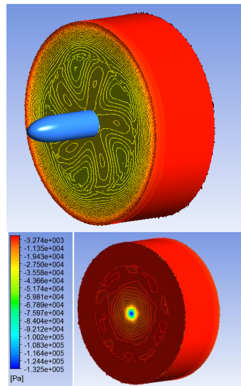
شکل ۱۴ سطح کیرشهف حول داکت و پروانه و توزیع فشار روی آن از دو نمای مشاهده.
