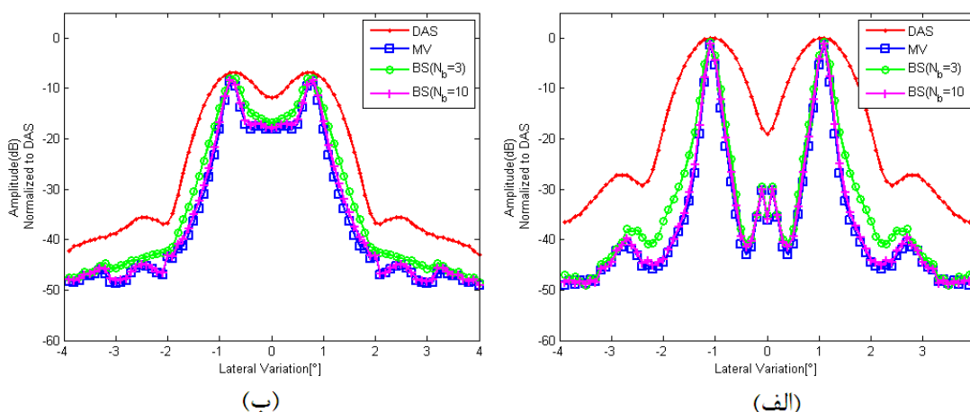
شکل ۳ تغییرات زاویه برای پرتو دیسگرهای (شکل دهنده های) پرتو مختلف. (الف) در عمق ۴۰ میلی متری، (ب) در عمق ۶۰ میلی متری.
