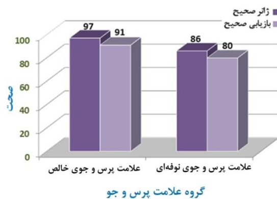
شکل ۵ نتایج سامانه پیشنهادی در عمق بازیابی ۱ برای فاصله اقلیدسی.
