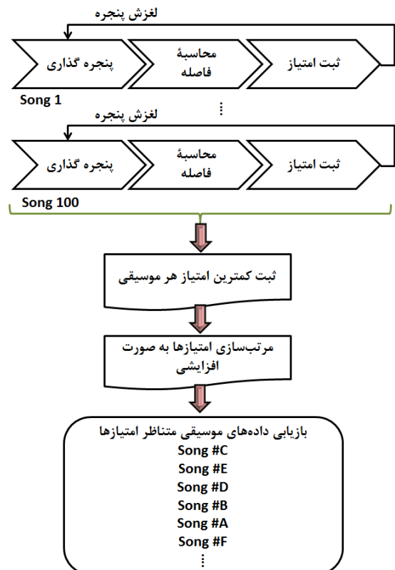
شکل ۴ روندنمای بلوک تطبیق - بازیابی.
