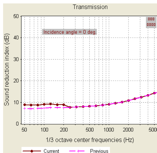
شکل ۴ شاخص افت تراگسیل امواج صوتی یک لایه‌ی خل‌دار (متخلخل) نوع میشل که به یک دیواره‌ی صلب نصب شده، برای درصدهای تخلخل ۹۵ درصد (منحنی خط‌چین) و ۴۵ درصد (منحنی پر رنگ) مقایسه شده‌اند.
