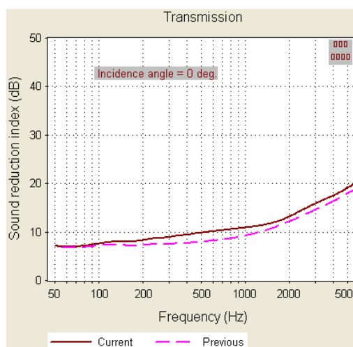
شکل ۶ شاخص افت تراگسیل صوتی یک لایه‌ی خل‌دار (متخلخل) نوع آتن‌برو که به یک دیواره‌ی صلب نصب شده، برای درصدهای تخلخل ۹۵ درصد (منحنی خط‌چین) و ۵۵ درصد (منحنی پر رنگ) مقایسه شده‌اند.
