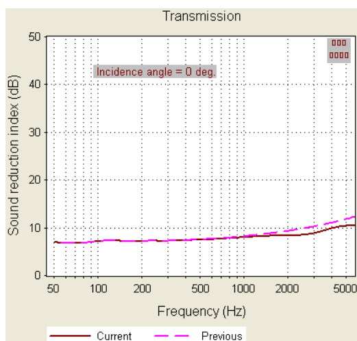
شکل ۴ شاخص افت تراگسیل امواج صوتی یک لایه‌ی خل‌دار (متخلخل) نوع آن‌برو که به یک دیواره‌ی صلب نصب شده، برای درصدهای تخلخل ۹۵ درصد (منحنی خط‌چین) و ۵۵ درصد (منحنی پر رنگ) مقایسه شده‌اند.
