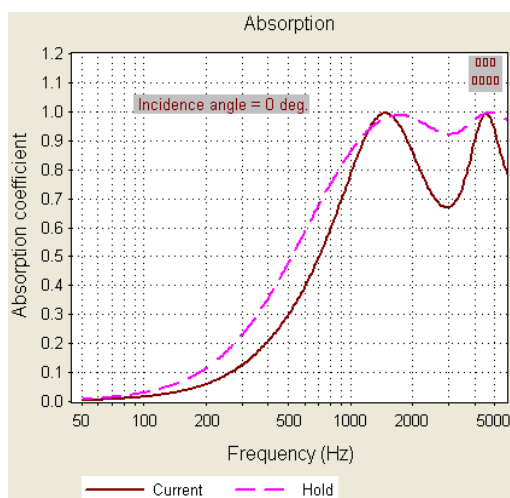
شکل ۳ میزان ضریب جذب یک لایه‌ی خل‌دار (متخلخل) نوع آن‌برو که به یک دیواره‌ی صلب نصب شده، برای درصدهای تخلخل ۹۵ درصد (منحنی خط‌چین) و ۵۵ درصد (منحنی پر رنگ) مقایسه شده‌اند.
