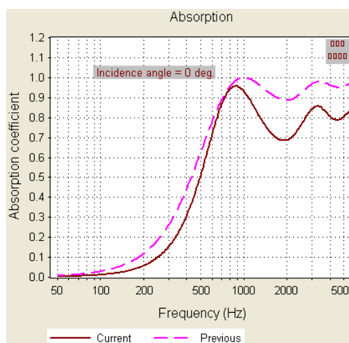
شکل ۵ ضریب جذب یک لایه‌ی خل‌دار (متخلخل) نوع آتن‌برو که به یک دیواره‌ی صلب نصب شده، برای درصدهای تخلخل ۹۵ درصد (منحنی خط‌چین) و ۴۵ درصد (منحنی پر رنگ) مقایسه شده‌اند.
