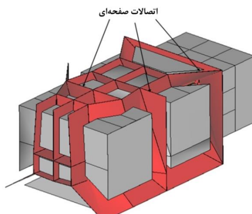
شکل ۶ اتصالات بین زیرسامانه‌ها در الگوی اِس‌ای‌ای خودرو.
