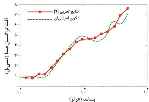
شکل ۱۰ مقایسه‌ی روش اِس‌اِی‌ای با نتایج آزمایشگاهی.
