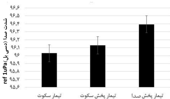
شکل ۸ مقادیر شدت صدای ثبت‌شده برای هریک از تیمارهای سکوت (صدای زمینه) بلندگو خاموش، پخش سکوت (پخش صدای زمینه) بلندگو روشن، پخش صدای افزایش‌یافته بلندگو روشن نشان داده‌شده‌اند. مقادیر متفاوت a و b بیانگر تفاوت معنی‌داری است.
