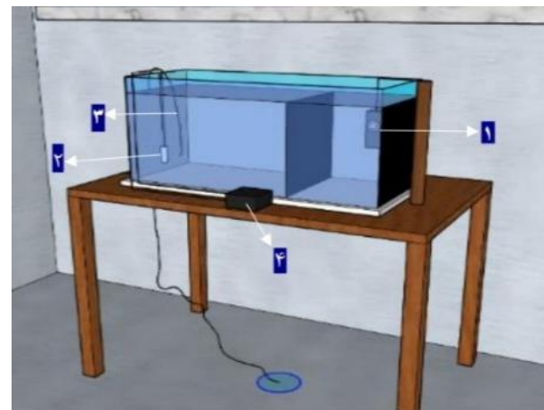
شکل ۱ نمای جانبی (کناری) از تانک آزمایشی مورد استفاده در این مطالعه و تجهیزات به‌کاررفته جهت سنجش و اندازه‌گیری صدا. (۱). گوینده جی بی ال؛ ۲. هیدروفون؛ ۳. سیم زمین و اتصالات؛ ۴. ضبط‌کننده صدا)
