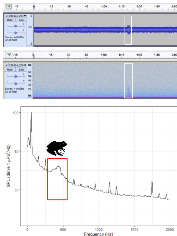
شکل ۳ تصویری از صداگستره منطقه نمونه‌برداری. (الف) اوسیلوگرام نوسان‌نگاره صوتی (ب) اسپکتروگرام طیف‌نگاره صوتی و (ج) تراکم طیف انرژی صوتی نمونه فیل ضبط‌شده نشان‌دهنده صداگستره در استخر نمونه‌برداری. کادرهای سفید در شکل‌های الف و ب نشان‌دهنده زمان وقوع صوت با منشاء زیستی می‌باشند. کادر قرمز رنگ شکل ج نشان‌دهنده افزایش شدت صوت در دامنه بسامدی ۴۰۰ تا ۵۰۰ هرتز مرتبط با اصوات تولیدشده با منشاء زیستی را نشان می‌دهد. در شکل ج، محور افقی دامنه بسامدهای صوتی و محور عمودی واحد سطح صوت را نشان می‌دهد.
