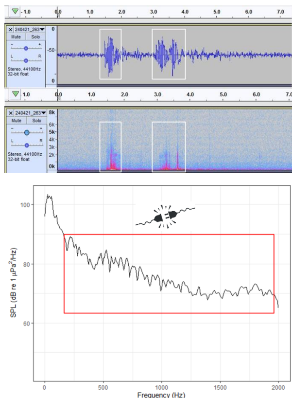
شکل ۴ تصویری از اضافه شدن منبع صوتی ثانویه ناشی از خطای در حین نمونه‌برداری نشان داده شده است. (شکل الف و ب) به ترتیب نوسان‌نگاره صوتی و طیف‌نگاره صوتی می‌باشند. کادرهای سفید نشان‌دهنده شکل نوسان و تغییرات انرژی در واحد زمان می‌باشند. (شکل ج) تراکم طیف انرژی صوتی فیل ضبط‌شده و کادر قرمز افزایش شدت ترازهای فشار صوتی در دامنه بسامدهای مختلف ناشی از خطای در حین نمونه‌برداری در دامنه بسامدهای ۱۲۵ تا ۲۰۰۰ هرتز قابل مشاهده است.
