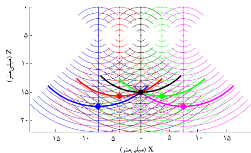
شکل ۲ مثالی از انتشار موج و خطوط تصویر پرتودیسگر (شکل‌دهنده پرتو) مرحله اول از پنج ارسال متفاوت [۱۵].
