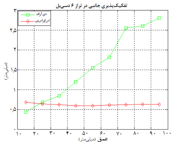
شکل ۹ تغییرات تفکیک پذیری (رزولوشن) جانبی بر حسب عمق در تراز ۶ دسی بل (براساس معیار فدا بل یو اچ ام) برای دو روش پرتودیسی (شکل دهی پرتو) دو مرحله ای و تمرکز ثابت در دریافت.
