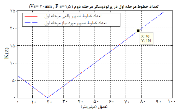
شکل ۱۰ نمودار K(z) بر حسب عمق تصویربرداری.
