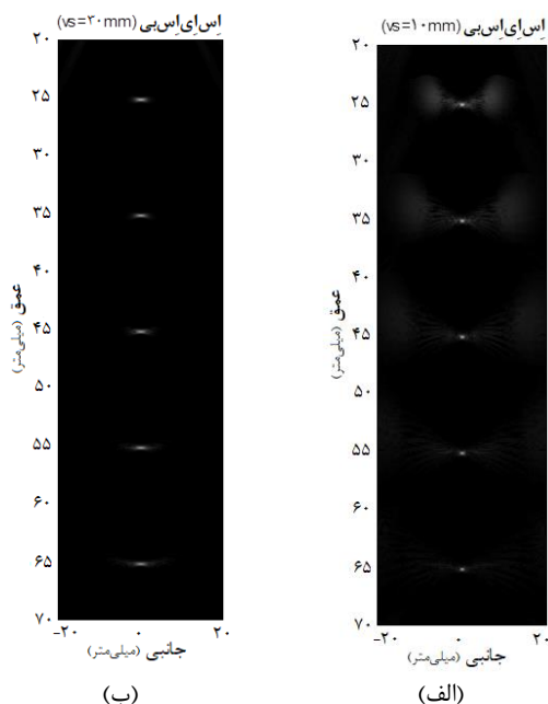
شکل ۷ تصویر فانتوم نقطه‌ای در روش پرتوديسي (شکل‌دهی پرتو) دو مرحله‌ای برای دو مقدار مختلف مربوط به عمق منبع مجازی (وی‌اس*). (الف) منبع مجازی در عمق ۱۰ میلی‌متری، (ب) منبع مجازی در عمق ۳۰ میلی‌متری. محدوده دینامیکی تصاویر ۶۰ دسی‌بل می‌باشد.
