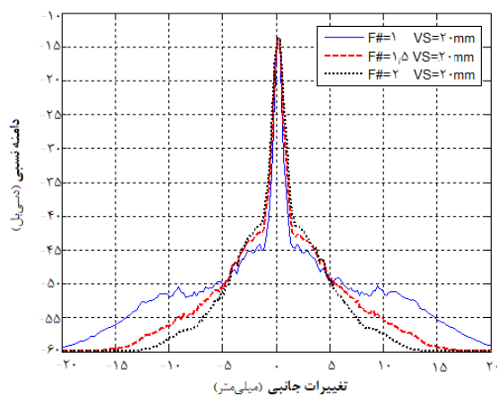
شکل ۹ تغییرات جانبی در عمق ۵۰ میلی‌متر برای سه مقدار مختلف F_{\#} .
