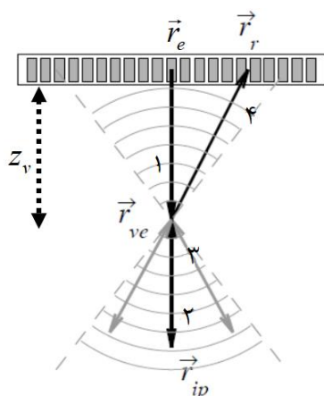
شکل ۱ مسافت طی شده توسط موج برای محاسبه تأخیر در پرتودیسگر (شکل‌دهنده پرتو) مرحله اول برای عنصر \vec{r}_r و نقطه تصویر \vec{r}_{ip} وقتی تمرکز ثابت در دریافت اعمال شده است [۱۵].
