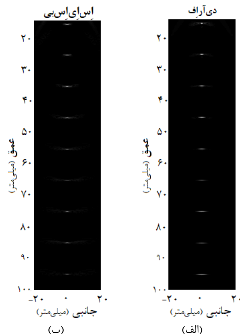
شکل ۸ (الف) روش تمرکز ثابت در دریافت، (ب) روش پرتودیسی (شکل دهی پرتو) دو مرحله‌ای با F_{\#} = 1.5 و منبع مجازی در عمق ۲۰ میلی‌متری. محدوده دینامیکی تصاویر ۶۰ دسی‌بل می‌باشد.
