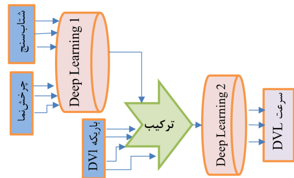
شکل ۴ ساختار شبکه عصبی.
