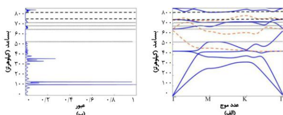
شکل ۱۲ (الف) نمودار ساختار باند شبکه بلور فونونی نیتريد بور برای پراکنده کننده‌های آب در بستر استیل به‌ازای r_1 = 0.4a_1 و r_2 = 0.2a_1 و (ب) طیف انتقال متناظر در راستای GM.
