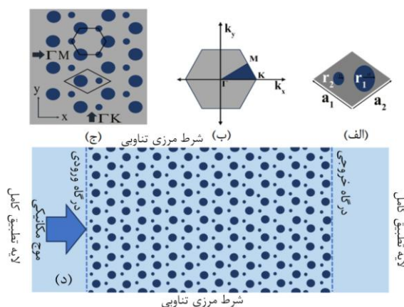
شکل ۱ (الف) طرح‌واره‌ای از شبکه نیتريد بور و سلول واحد آن، (ب) ناحیه بریلوین و ناحیه بریلوین تقلیل‌ناپذیر، (ج) جهت‌های موج ورودی و (د) طرح‌واره‌ای از ساختار نیتريد بور برای محاسبه طیف انتقال در جهت \Gamma M .
