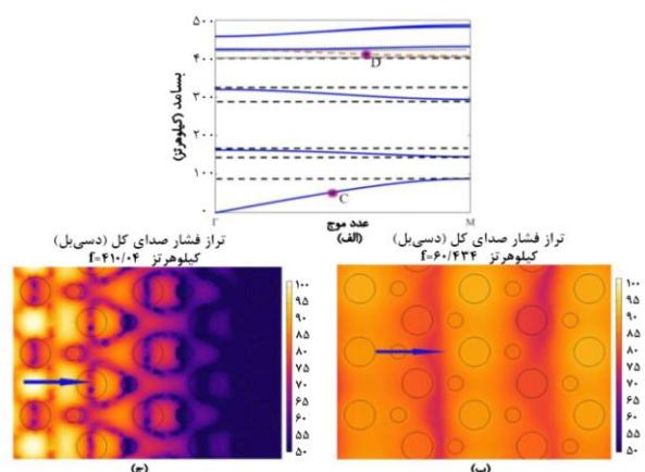
شکل ۱۰ (الف) ساختار باند در راستای FM، به همراه الگوی میدان در بسامدهای نمونه نشان داده شده با حروف C و D. (ب) و (ج) D.
