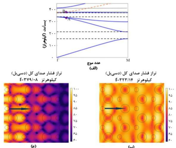
شکل ۴ (الف) ساختار باند در راستای GM، به همراه الگوی میدان در بسامدهای نمونه نشان داده شده با حروف A و B. (ج) B.
